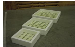
Søylefundament
