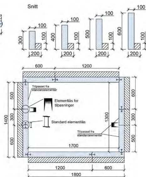
Som søylefundament
