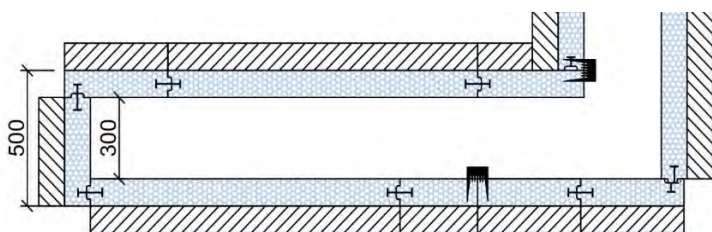
Som såleforskaling
